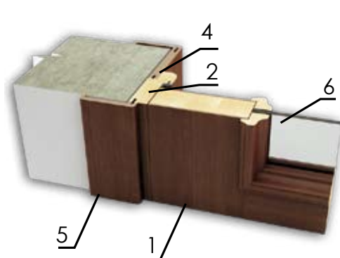
Разрез двери. Конструкция Door cross section. Design
