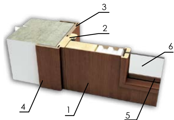
Разрез двери. Конструкция Door Cross Section. Design
