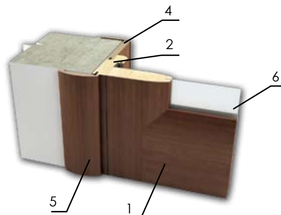
Разрез двери. Конструкция Door cross section. Design
