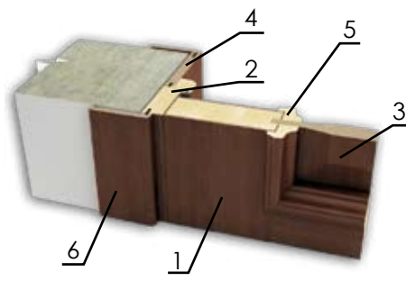
Разрез двери. Конструкция Door cross section. Design
