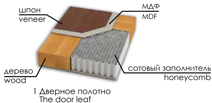
Разрез двери. Конструкция Door Cross Section. Design
