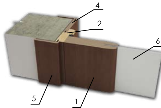
Разрез двери. Конструкция Door cross section. Design
