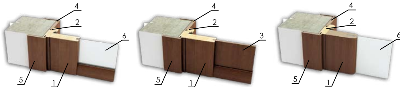
Разрез двери. Конструкция Door cross section. Design
